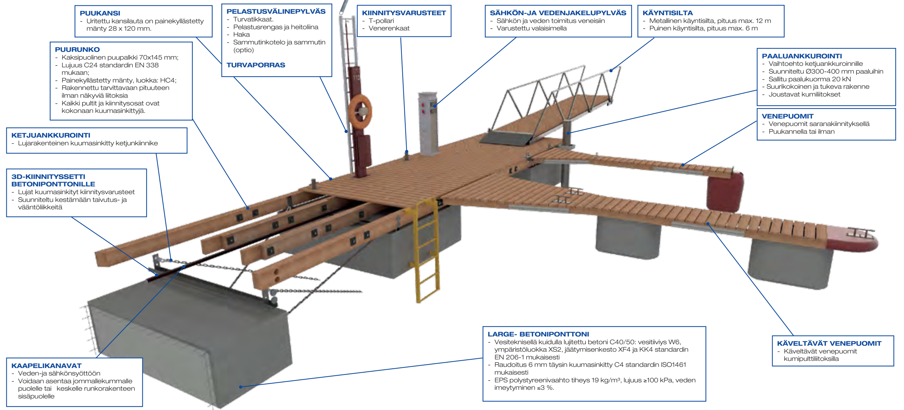
PÄÄTYLIITOS
